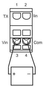
Voltage Input
